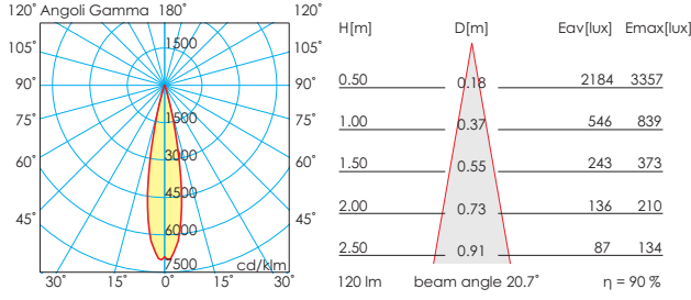
20° @350mA
