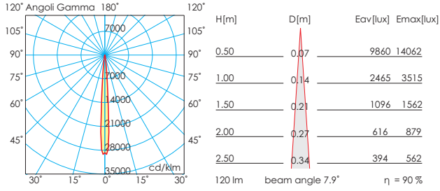
10° @350mA
